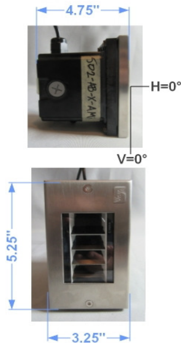
FIG. 1 LUMINAIRE
