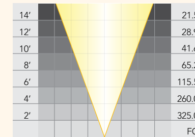
PAR 36 Halogen: LNH-50 WFL
