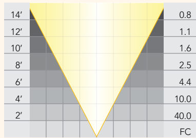
PAR 36: LN-25 VWFL
