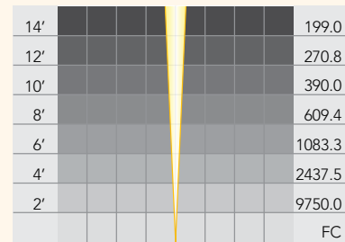
PAR 36 Halogen: LNH-50 VNSP
