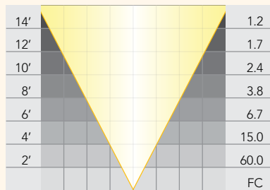
PAR 36: LN-50 VWFL
