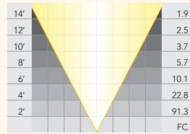
PAR 36 Halogen: LNH-7558
