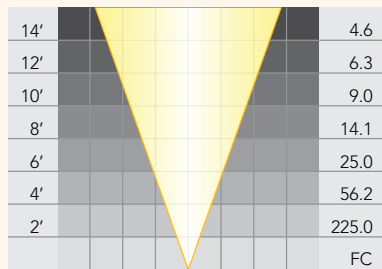
PAR 36: LN-50 WFL
