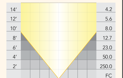
PAR 36 Halogen: LN-7606
