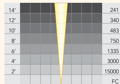
PAR 36 Halogen: LN-7600
