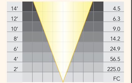
PAR 36 Halogen: LNH-35 WFL
