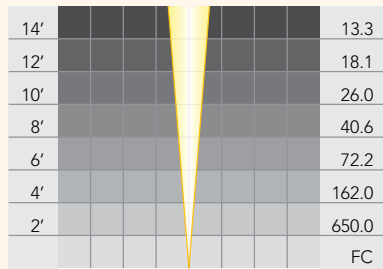
PAR 36: LN-25 NSP
