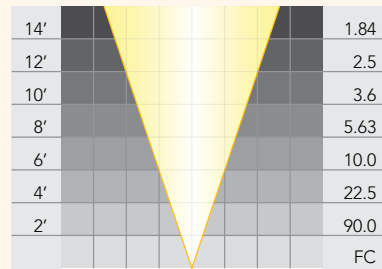
PAR 36: LN-25 WFL
