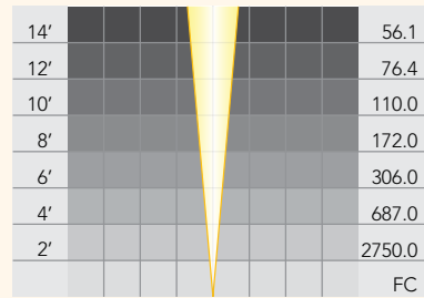
PAR 36: LN-50 NSP
