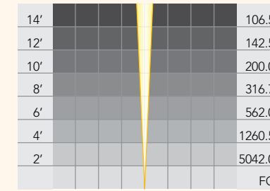
PAR 36 Halogen: LNH-35 VNSP
