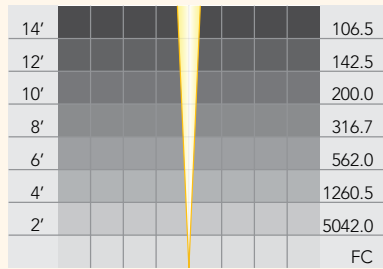
PAR 36: LN-50 VNSP
