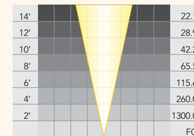
PAR 36 Halogen: LN-7610
